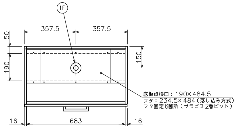
排水取り合い図
