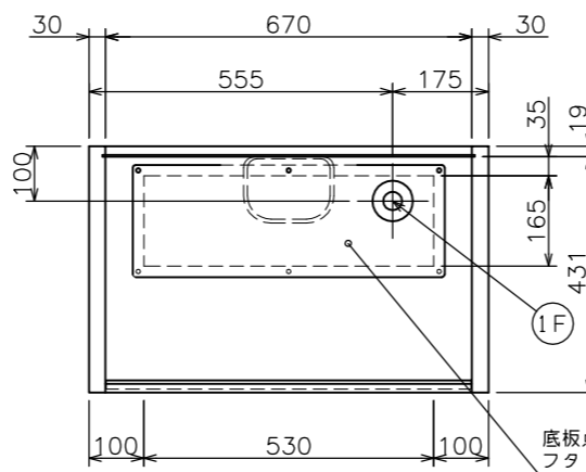
排水取り合い図
