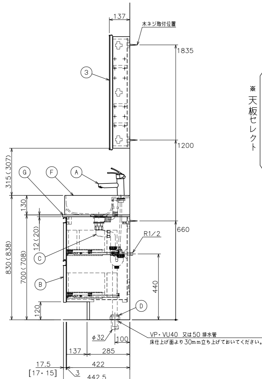
給・排水取り合い図
