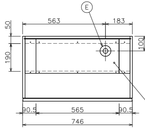
給・排水取り合い図
