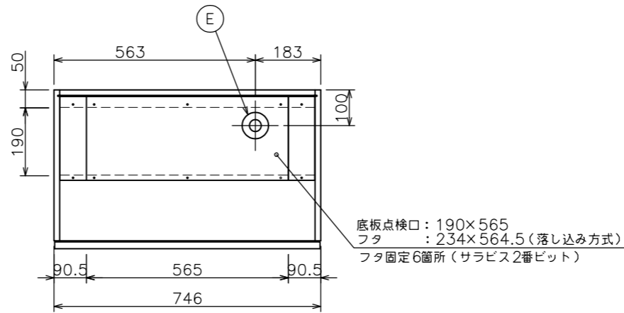
給・排水取り合い図
