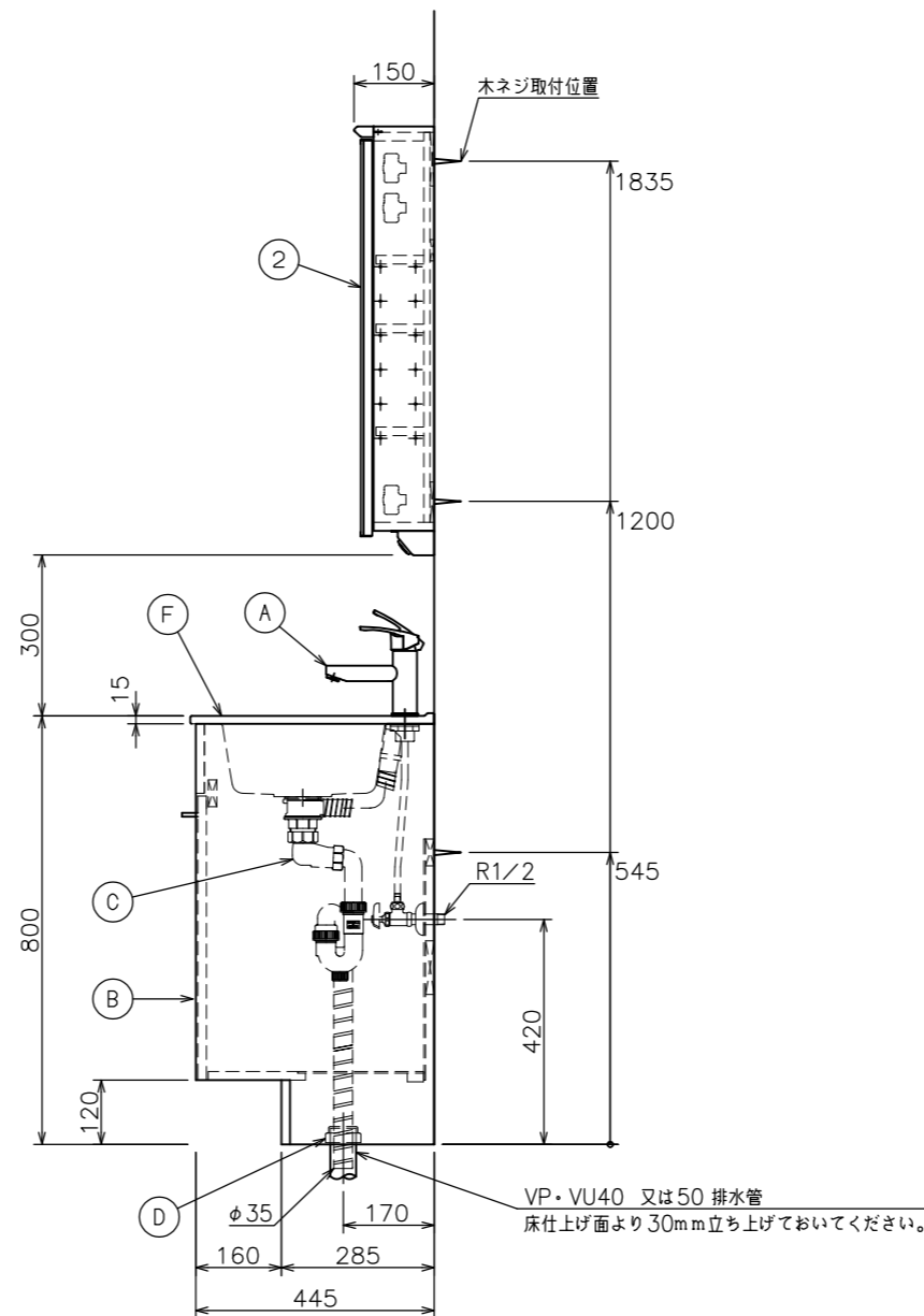
給・排水取り合い図
