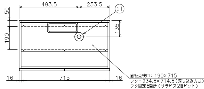
排水取り合い図
